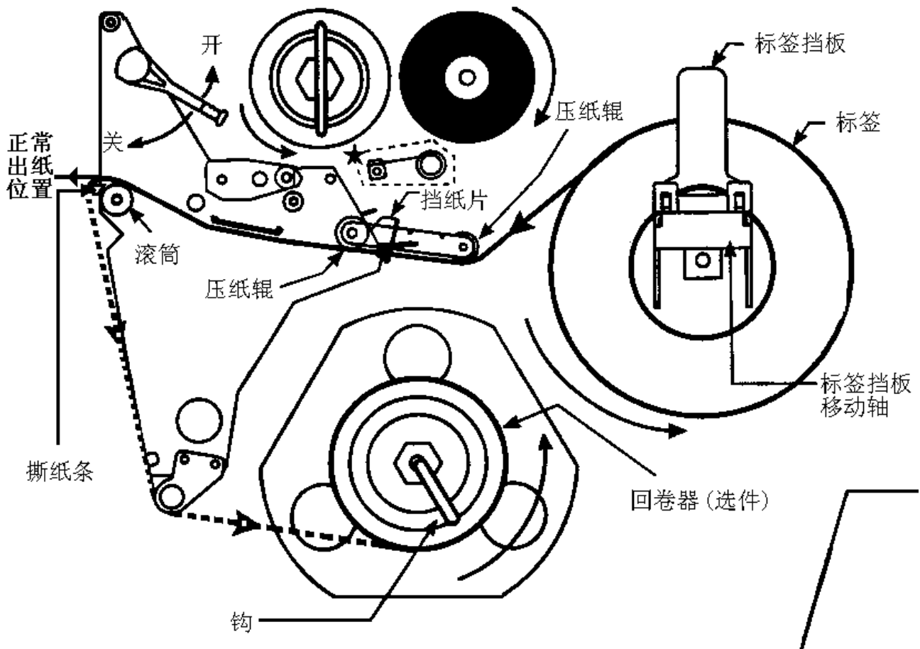
图 5 标签安装图
